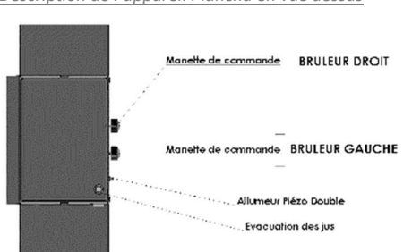
Description de l'appareil Plancha en vue dessus
